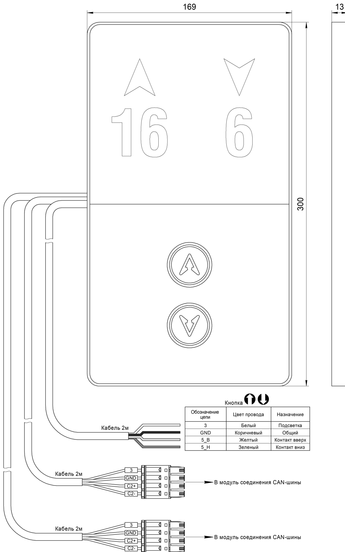
Рис.1 Внешний вид Вызывной пост ОНИКС НШЕК.468381.024
